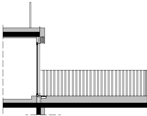
Schnitt 12/2
