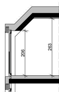
Schnitt 12/3
