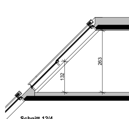
Schnitt 12/4
