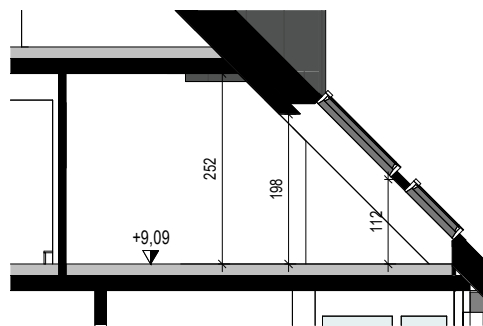
Schnitt 18.A
