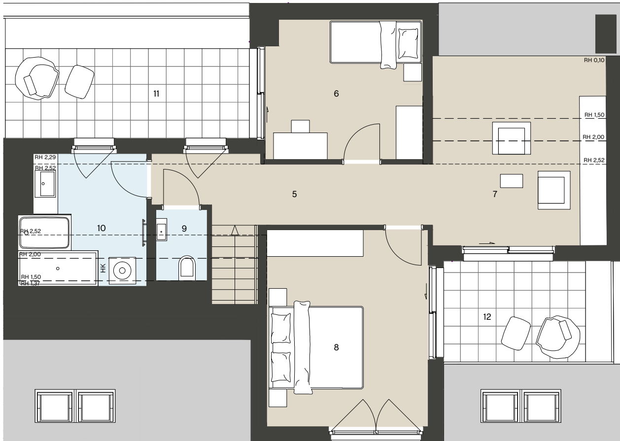
2. Dachgeschoss
