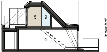
Schemaschnitt
