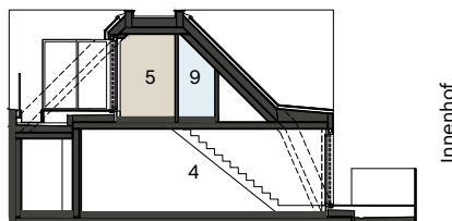
Schemaschnitt
