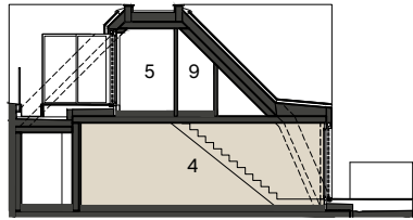
Schemaschnitt
