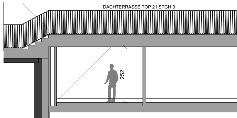
SCHNITT 3-3
