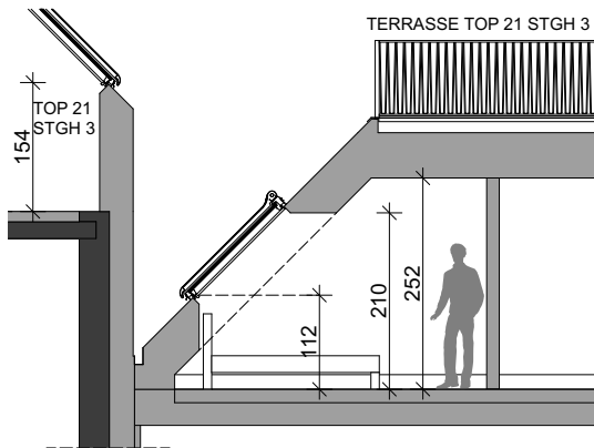
SCHNITT 2-2
