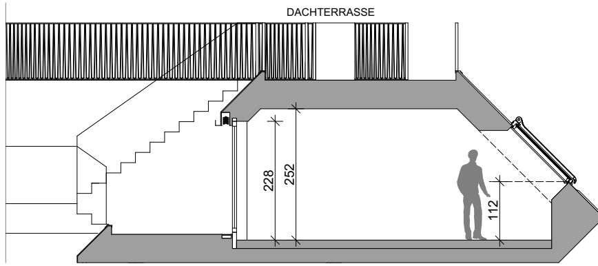
SCHNITT 1-1
