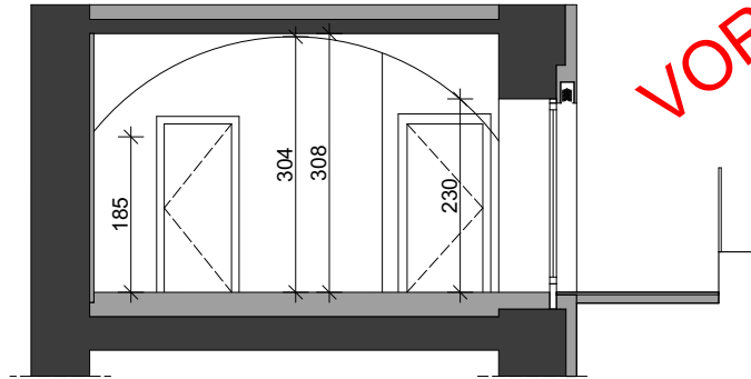
SCHNITT 1-1
