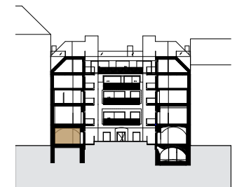
SCHNITT 3-3
