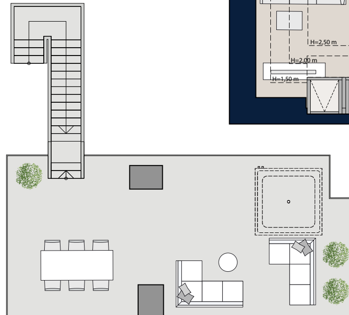
Dachterrasse
