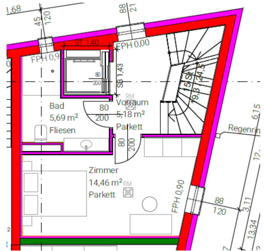
1.OG
